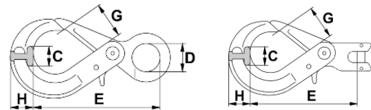
Crochet autobloquant à œil TWN 0798, classe 8
